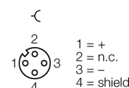
Подпись контактов
