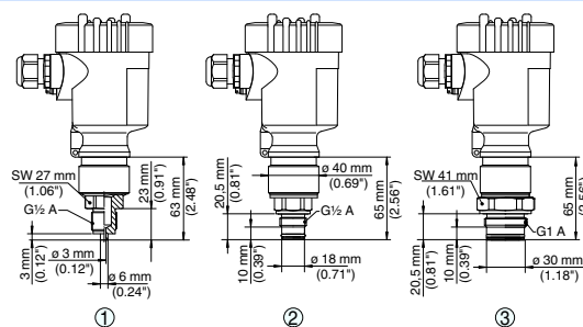
Размеры VEGABAR 53
