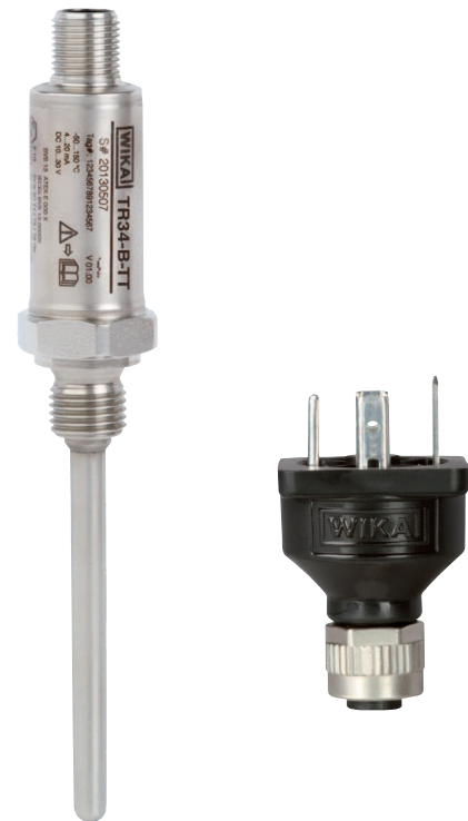
Рис. слева: термометр сопротивления, модель TR34 Рис. справа: адаптер M12 x 1 для углового разъема DIN EN 175301-803
